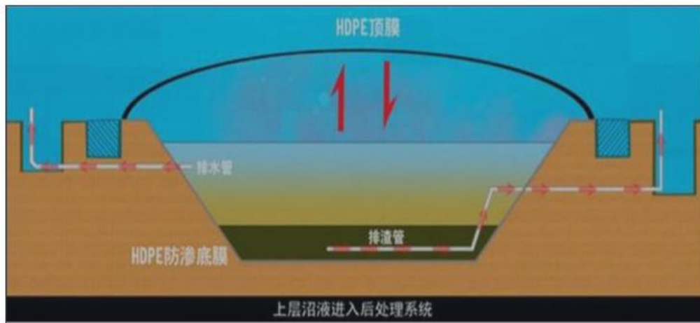
图 3-4 黑膜沼气池示意图
