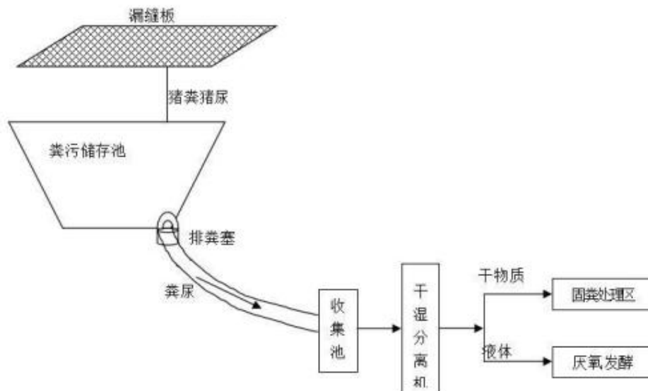
图 4-1 堆粪房处理流程图
