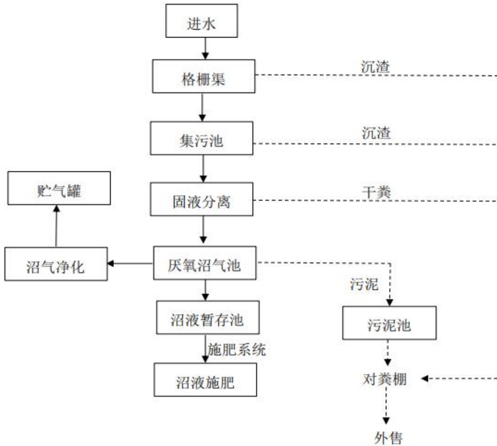
图 3-3 污水处理工艺流程图
