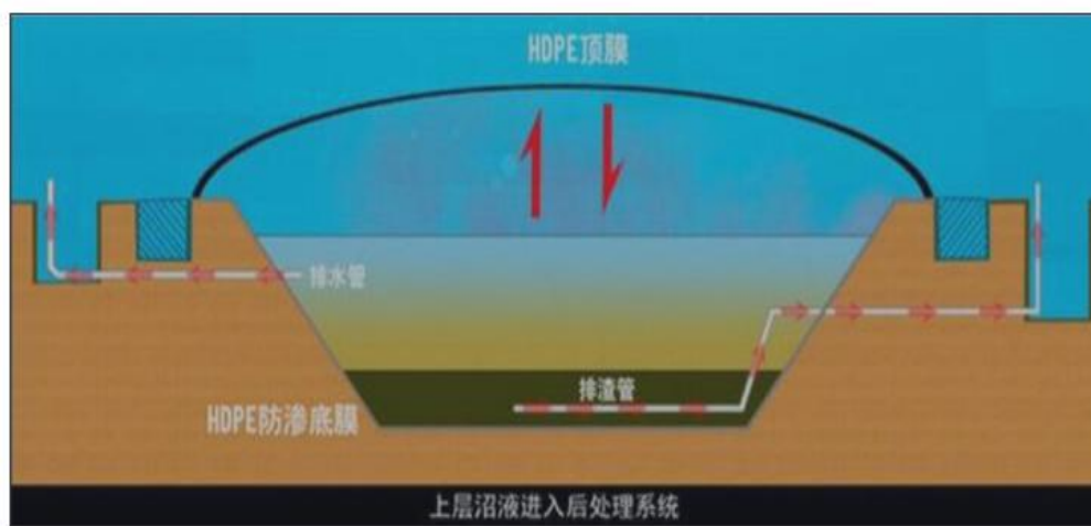
图3 黑膜沼气池示意图
