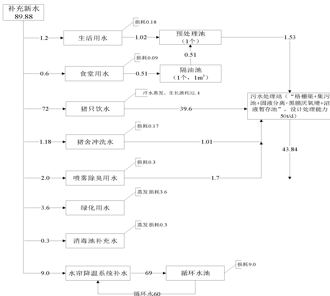
图 2.4-1 夏季全场水平衡图 (单位: m³/d)
