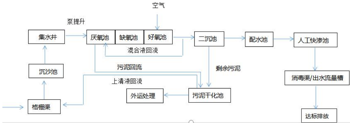
图 2-2 项目生产工艺及产污环节图
