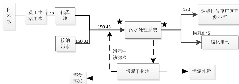
图 2-1 项目水平衡图 (m 3 /d) 监测点位：★
