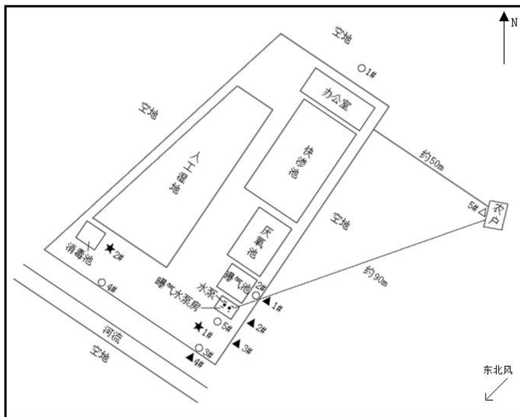
图 6-1 布点示意图 ●：噪声源 ▲：其他噪声检测点 △：敏感点噪声检测点 ★：废水检测点 ○：无组织排放废气检测点
