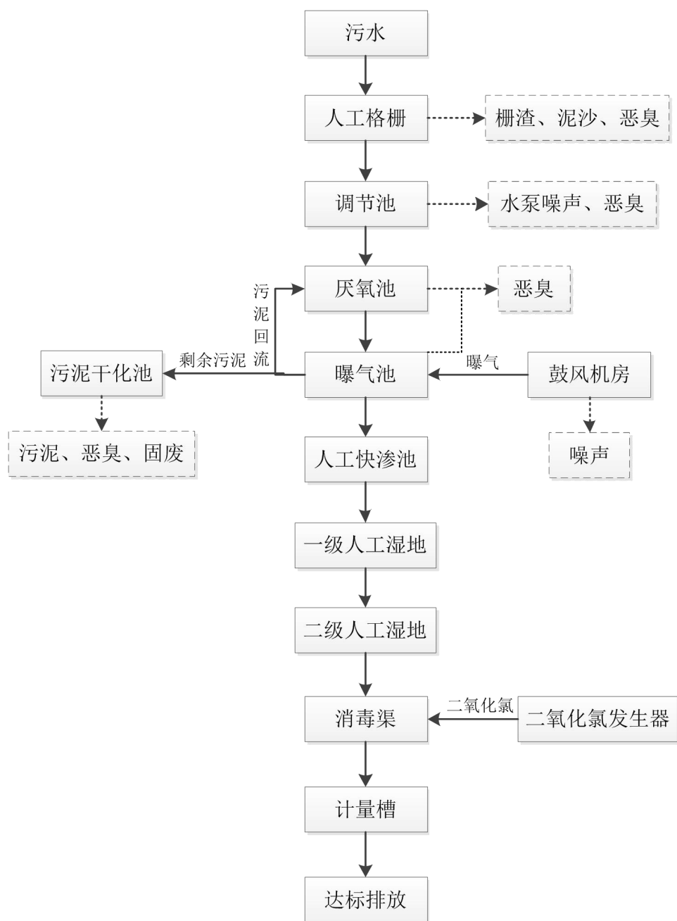
图 2-2 生产工艺流程图及产污位置图
